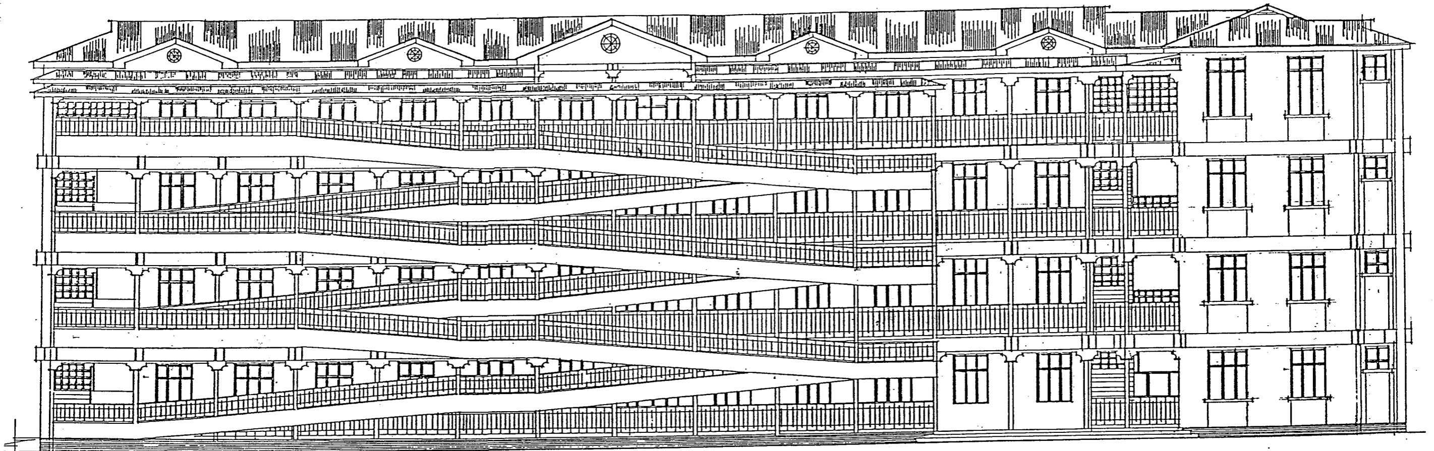
R · H · S ELEVATION 1:100
